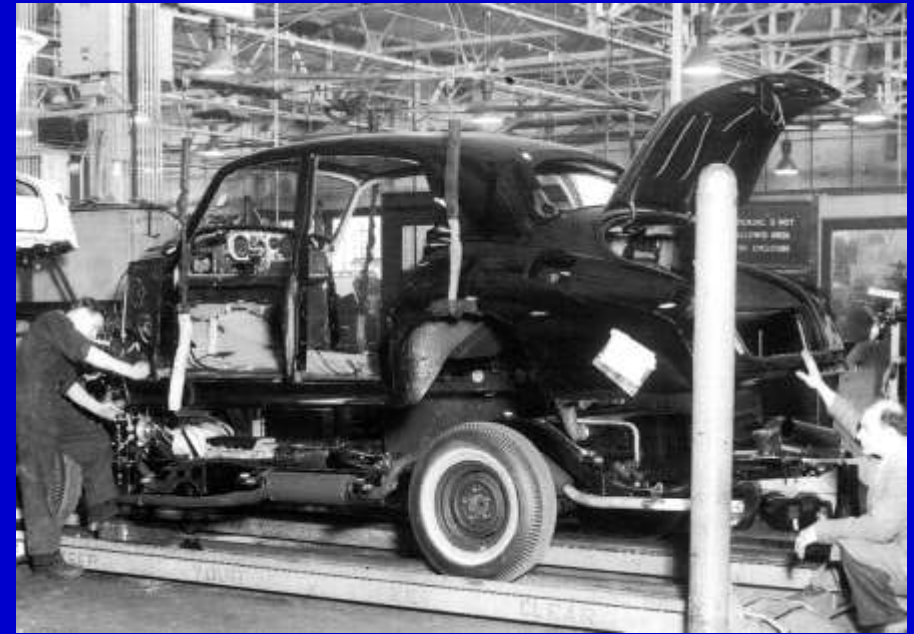
Absetzen der Karrosserie auf das Chassis
